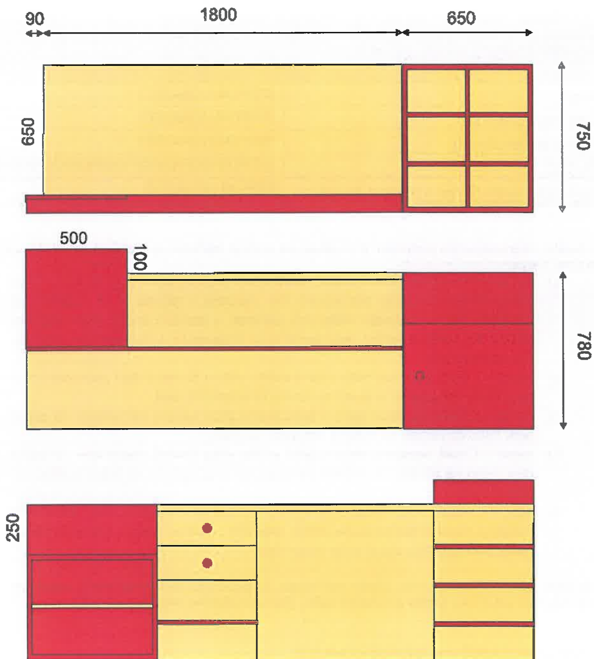
Hrabadlo - spodní nika - přední část s dvířka, zadní část police, přepažení uprostřed
